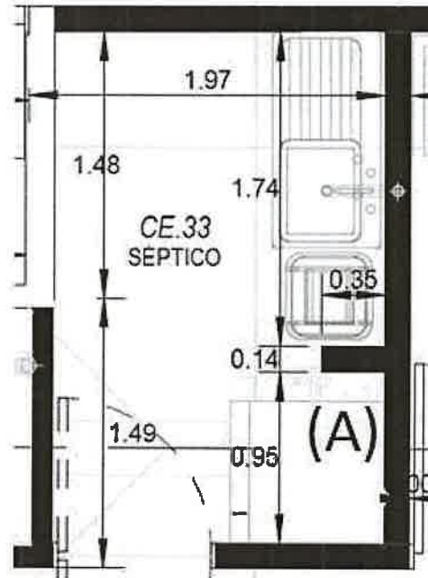
Ejemplo de Ubicación de Lavachatas, área disponible como (A)
