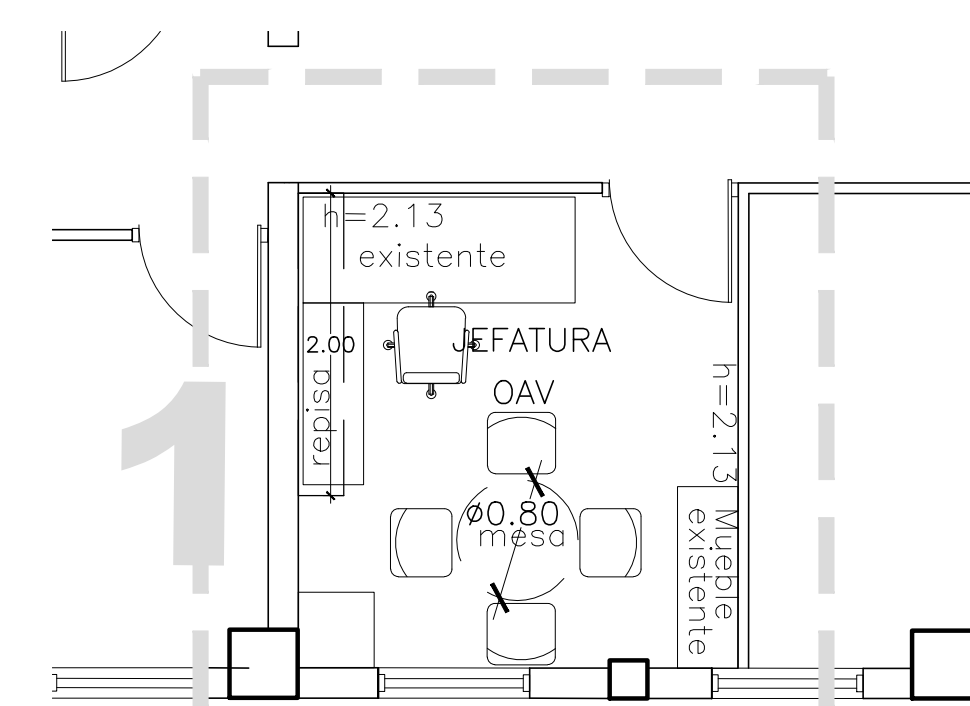
MUEBLE ACOTADO
