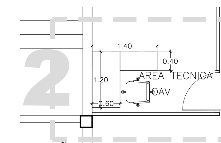
MUEBLE ACOTADO
