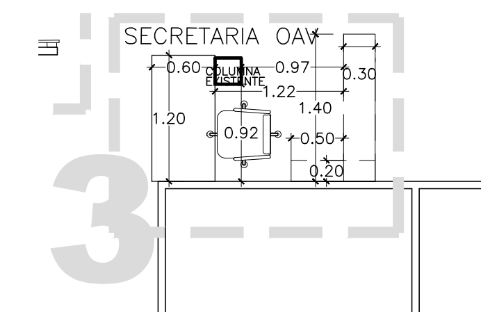
MUEBLE ACOTADO
