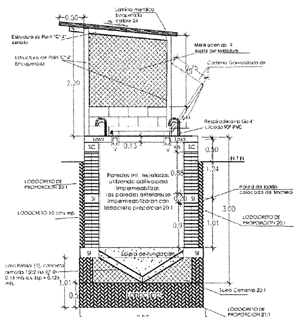
SECCION A-A CELDA DE DESECHOS BIOINFECCIOSOS ESC 1:50
