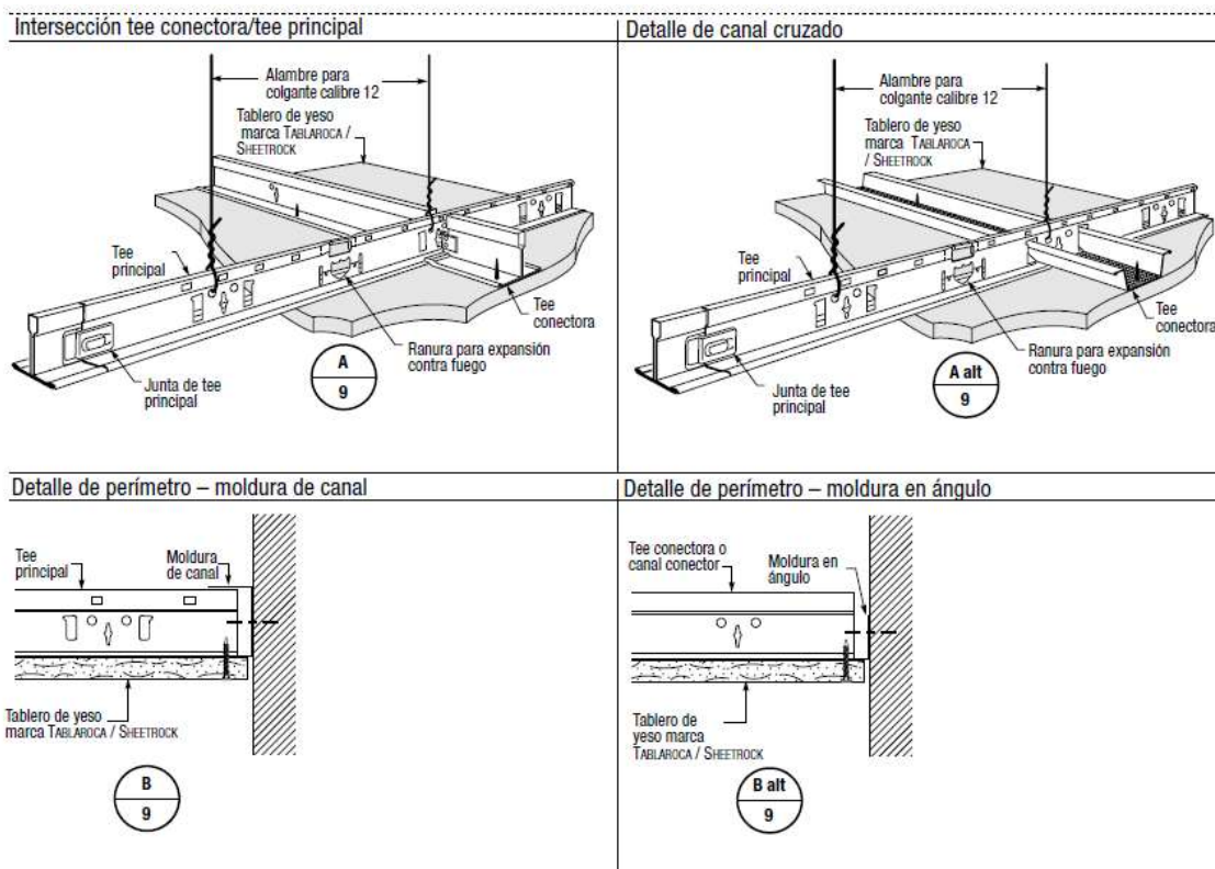
Figura. Suspensiones tipo para cielo de tablayeso
